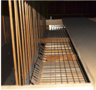
Mechanische Holzleisten zur Betätigung der Kegelladen.
